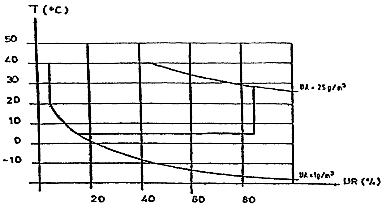
Fig. 2 Condizioni normali di prova
