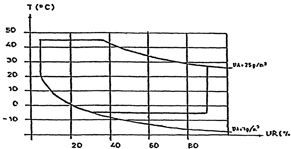
Fig. 3 Condizioni estreme di prova
