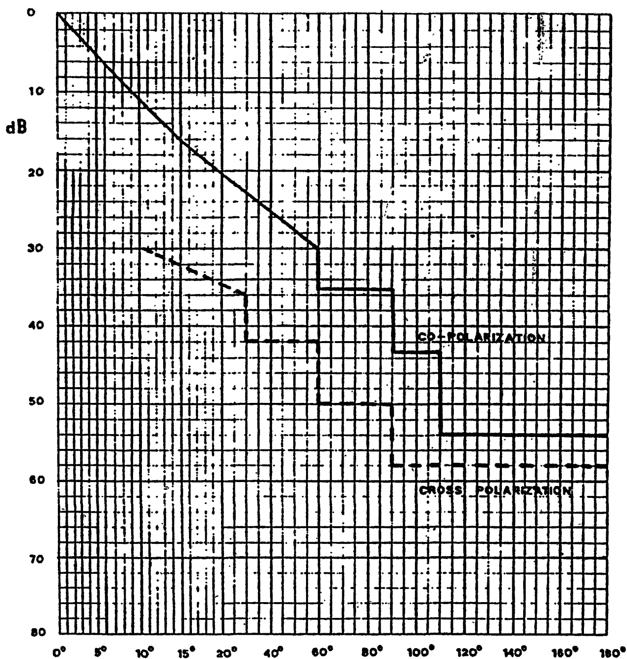
FIG:5 maschera del diagramma di radiazione azimutale di antenna
