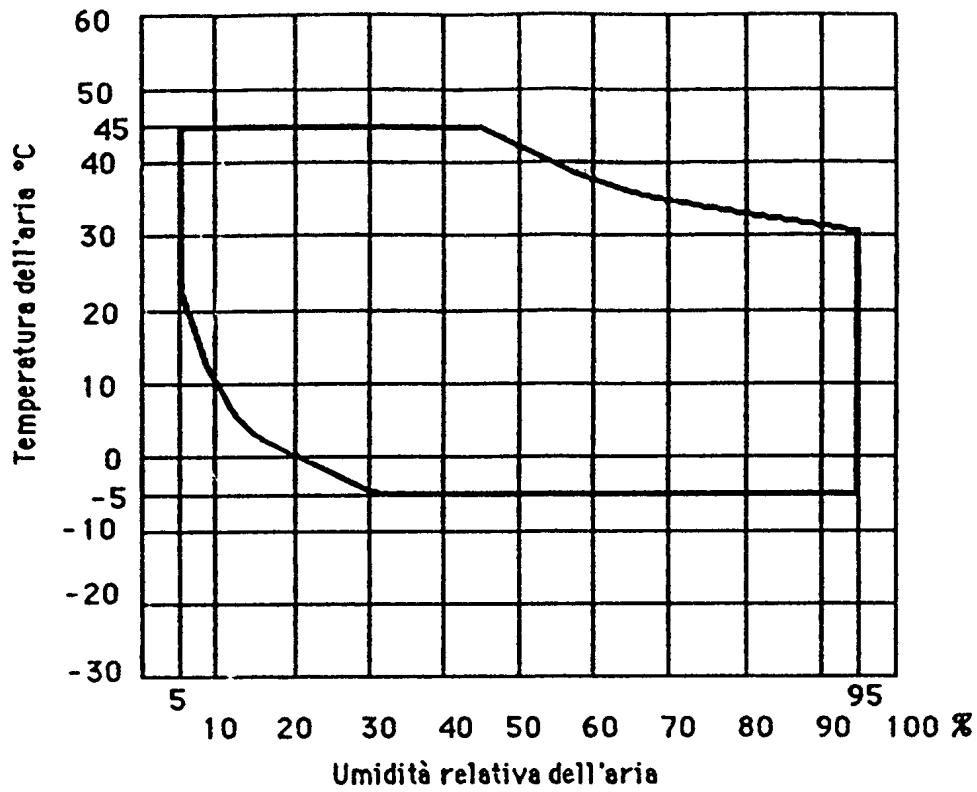
FIGURA 1 : CLIMATOGRAMMA PER LE PROVE AMBIENTALI
