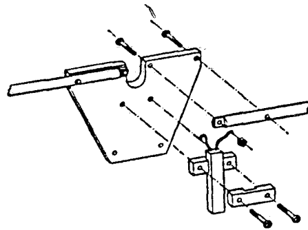
Vista parzialmente esplosa
