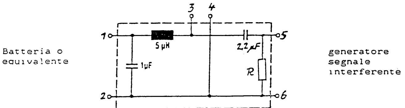
Fig. 19-a. Filtro di rete.
