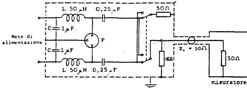
Fig. 4 - Esempio di rete normalizzata a V ( 50 \Omega , 50 \mu H ).
