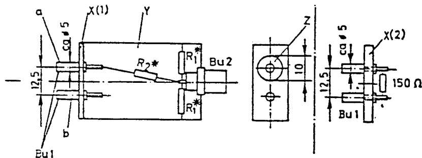
Fig. 35. Adattatore.
