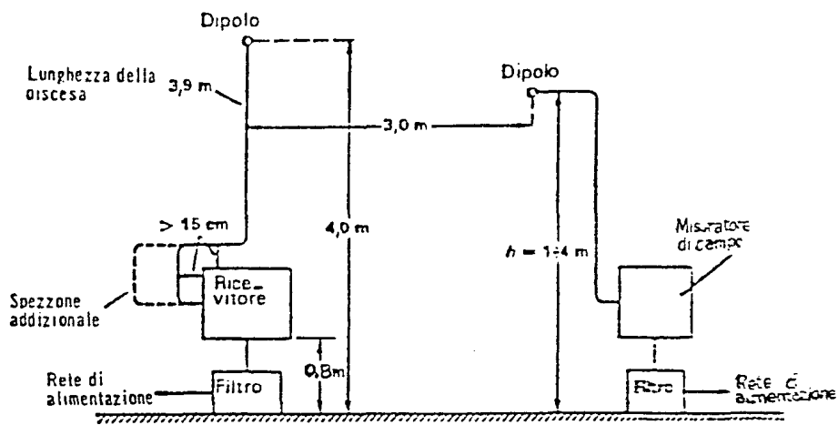
Fig. 7 - Misura all'aperto a 3 m di distanza
