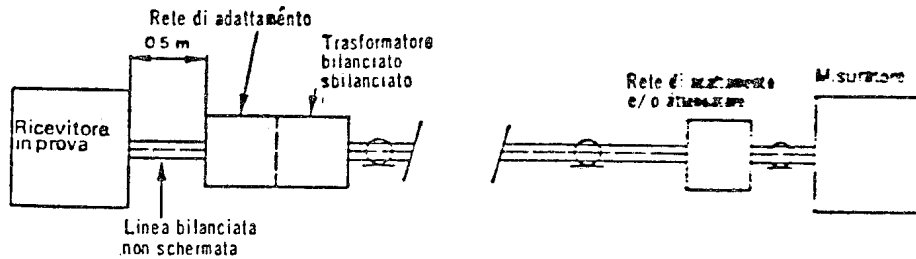
Fig. 11 - Disposizione degli elementi per la misura su un ricevitore con entrata d'antenna bilanciata.
