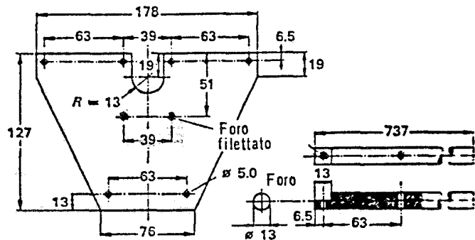
Sostegno del dipolo (metacrilato di metile di 6 mm di spessore)
