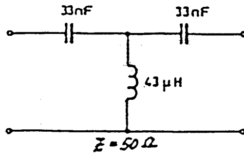
Fig. 20. Filtro passa-alto, 100 KHz.
