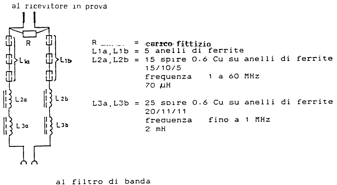
Fig. 29. Filtro per altoparlante.
