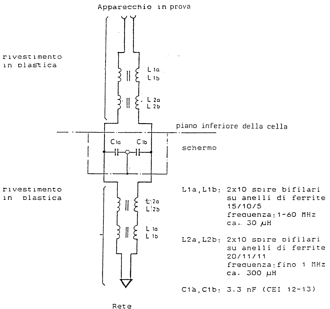
Fig. 28. Filtro rete.
