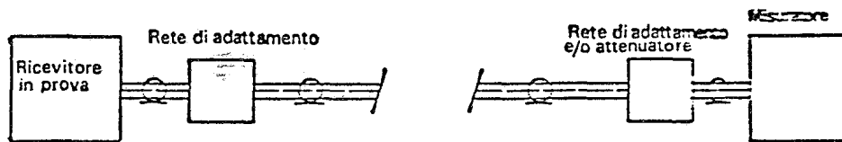
Fig. 10 - Disposizione degli elementi per la misura su un ricevitore con entrata di antenna entrata di antenna coassiale.
